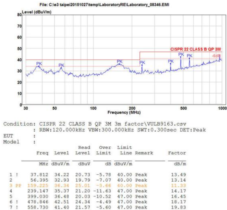
图 5-6 RE 测试垂直方向
