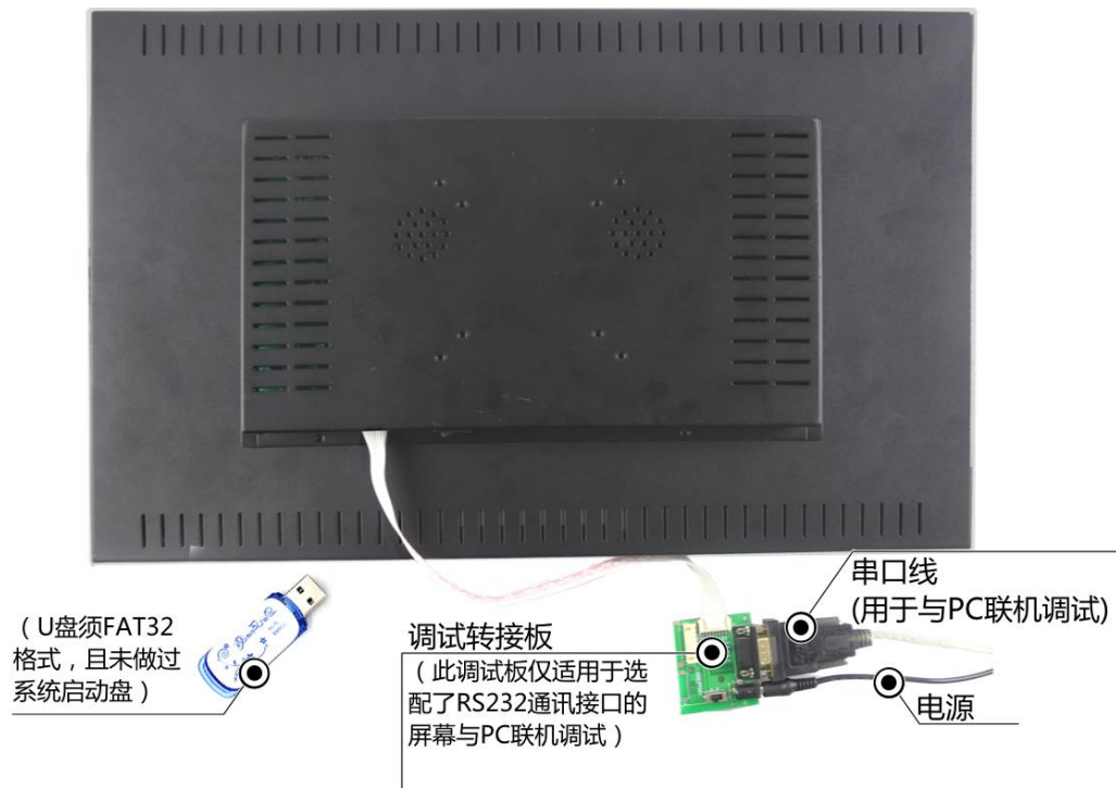
图 1-3 调试工具图
