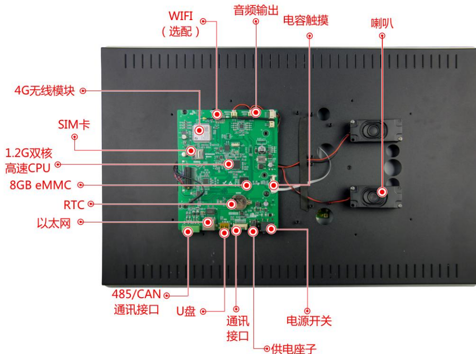
图 1-2 硬件配置图
